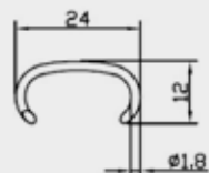
ANELLATRICE PNEUMATICA TC7C
