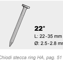
Chiodi stecca ring HA, pag. 51
